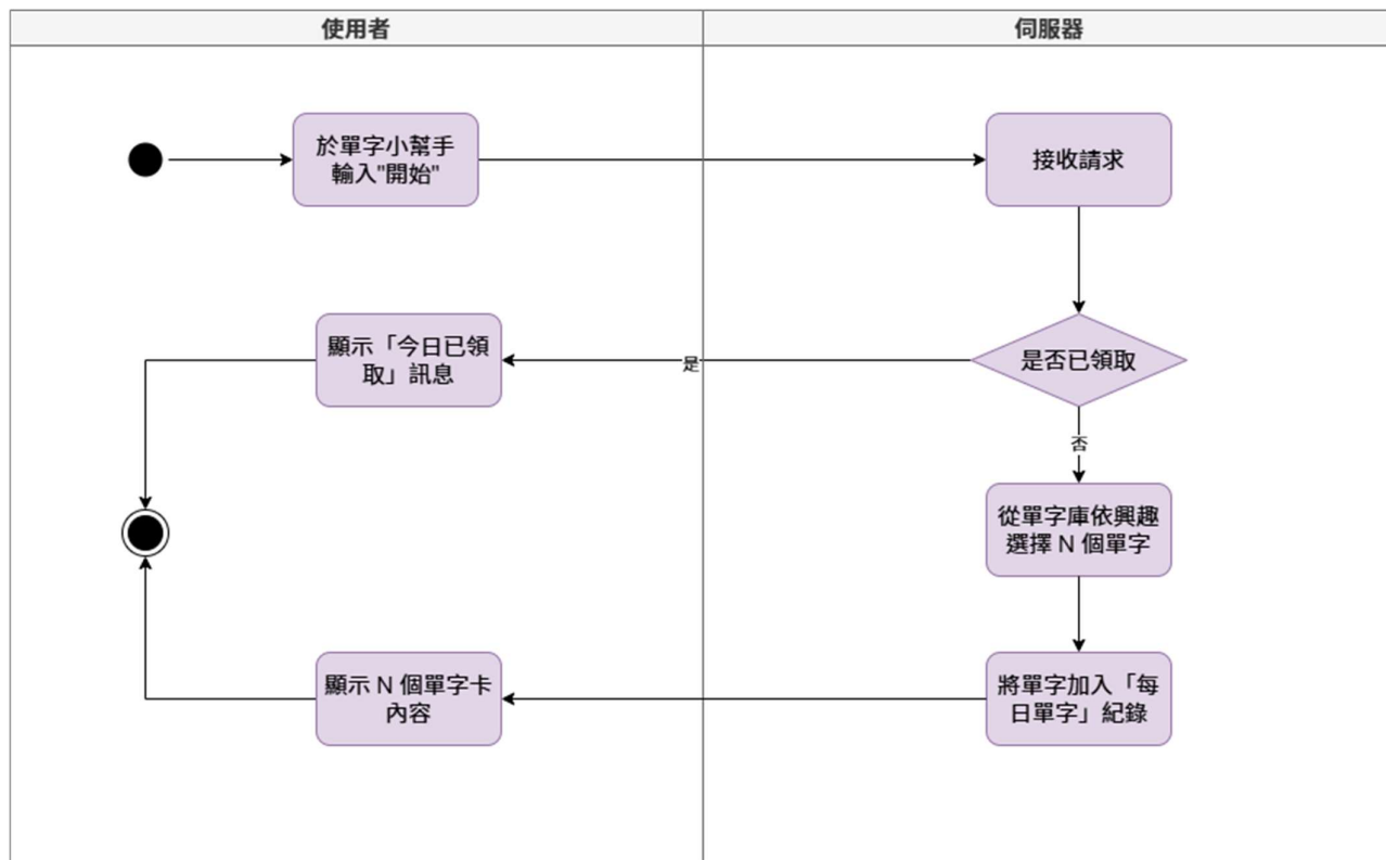
圖 5-3-10 領取單字卡之活動圖
