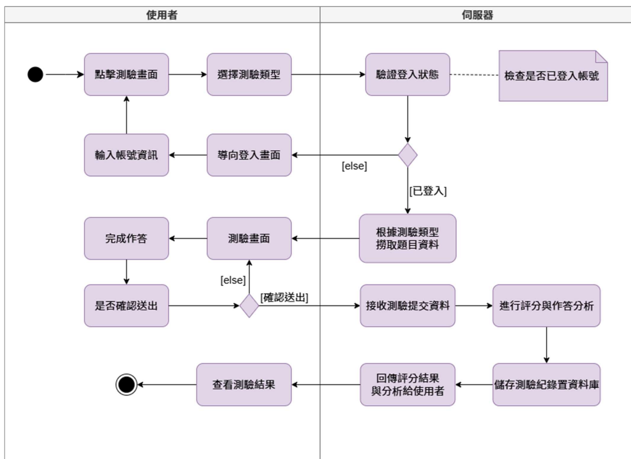
圖 5-3-5 測驗之活動圖
