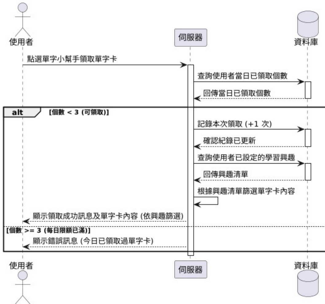
圖 6-1-9 領取單字卡之循序圖
