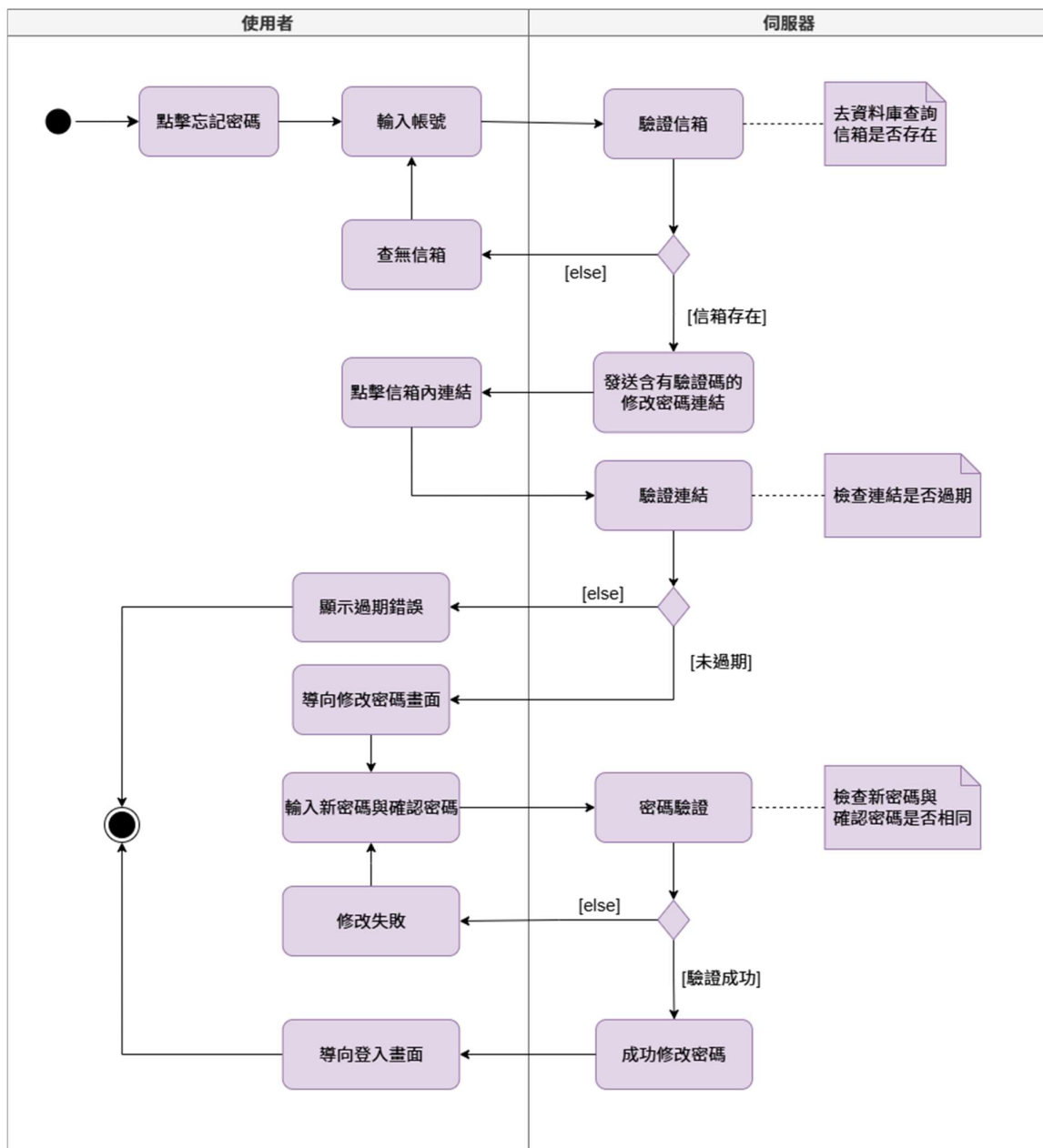
圖 5-3-3 忘記密碼之活動圖
