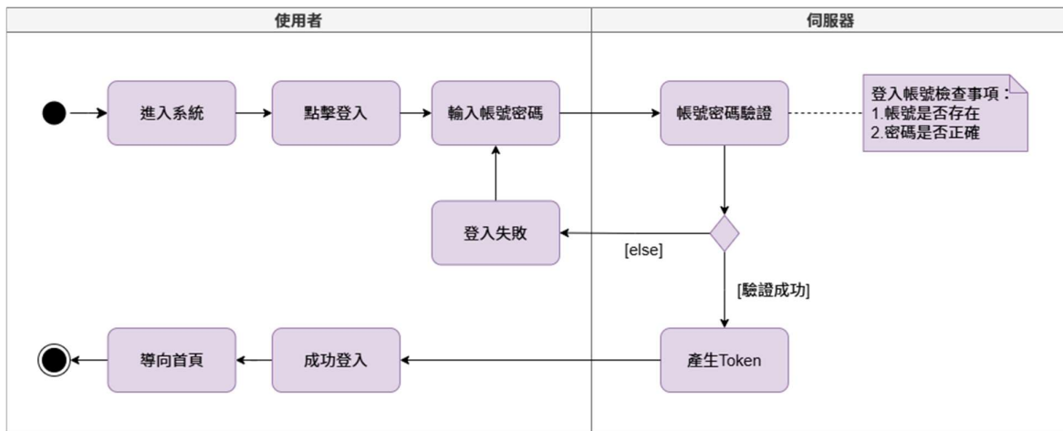
圖 5-3-2 登入之活動圖
