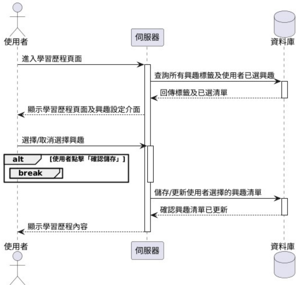
圖 6-1-11 選擇興趣之循序圖
