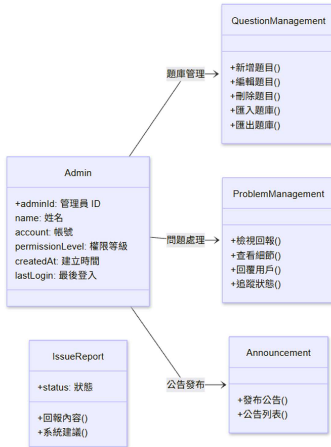
圖 5-4-3 管理與問題回報之類別圖
