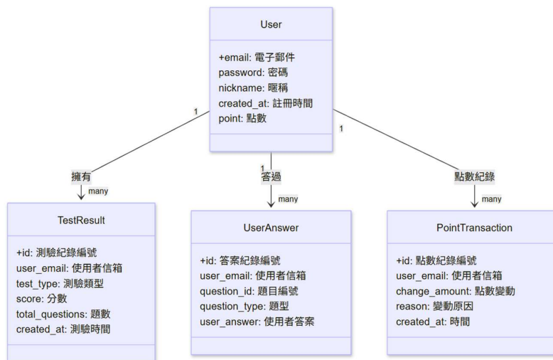
圖 5-4-2 使用者與基本測驗記錄之類別圖
