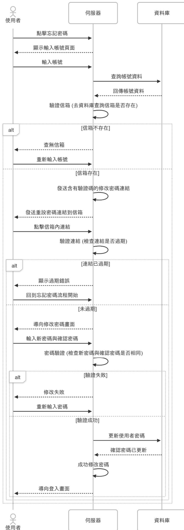
圖 6-1-3 忘記密碼之循序圖
