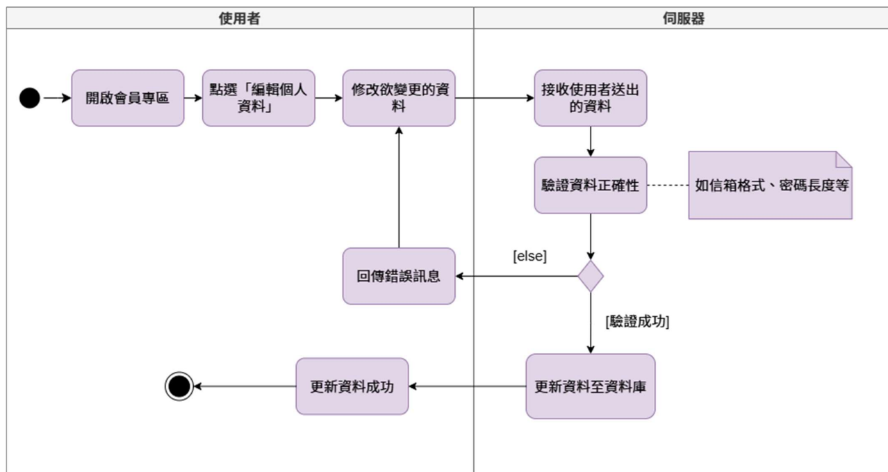
圖 5-3-8 使用者編輯個人資料之活動圖
