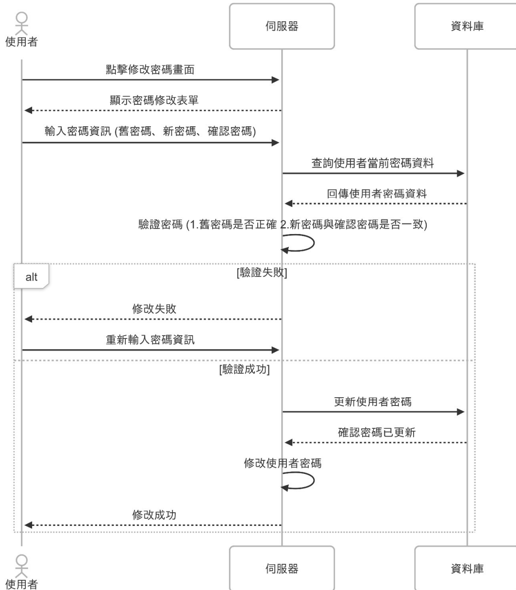
圖 6-1-4 修改密碼之循序圖
