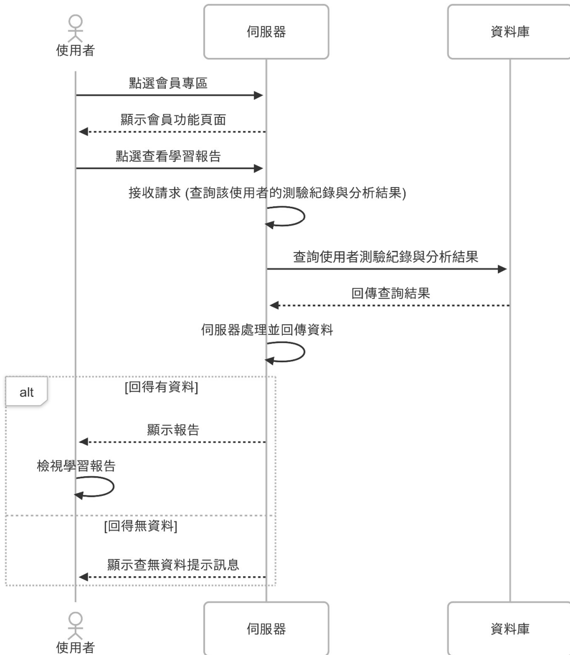
圖 6-1-6 查看學習報告之循序圖
