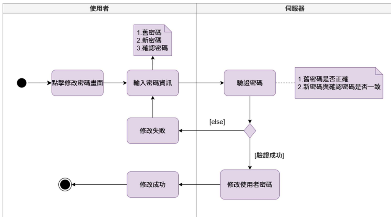
圖 5-3-4 修改密碼之活動圖
