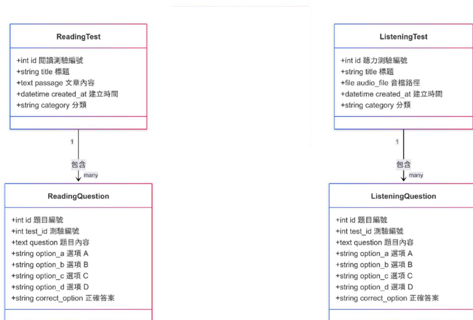
圖 5-4-4 測驗之類別圖
