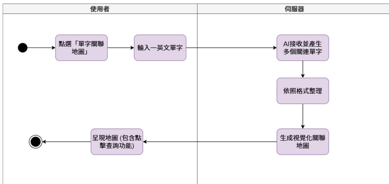
圖 5-3-9 單字關聯地圖之活動圖
