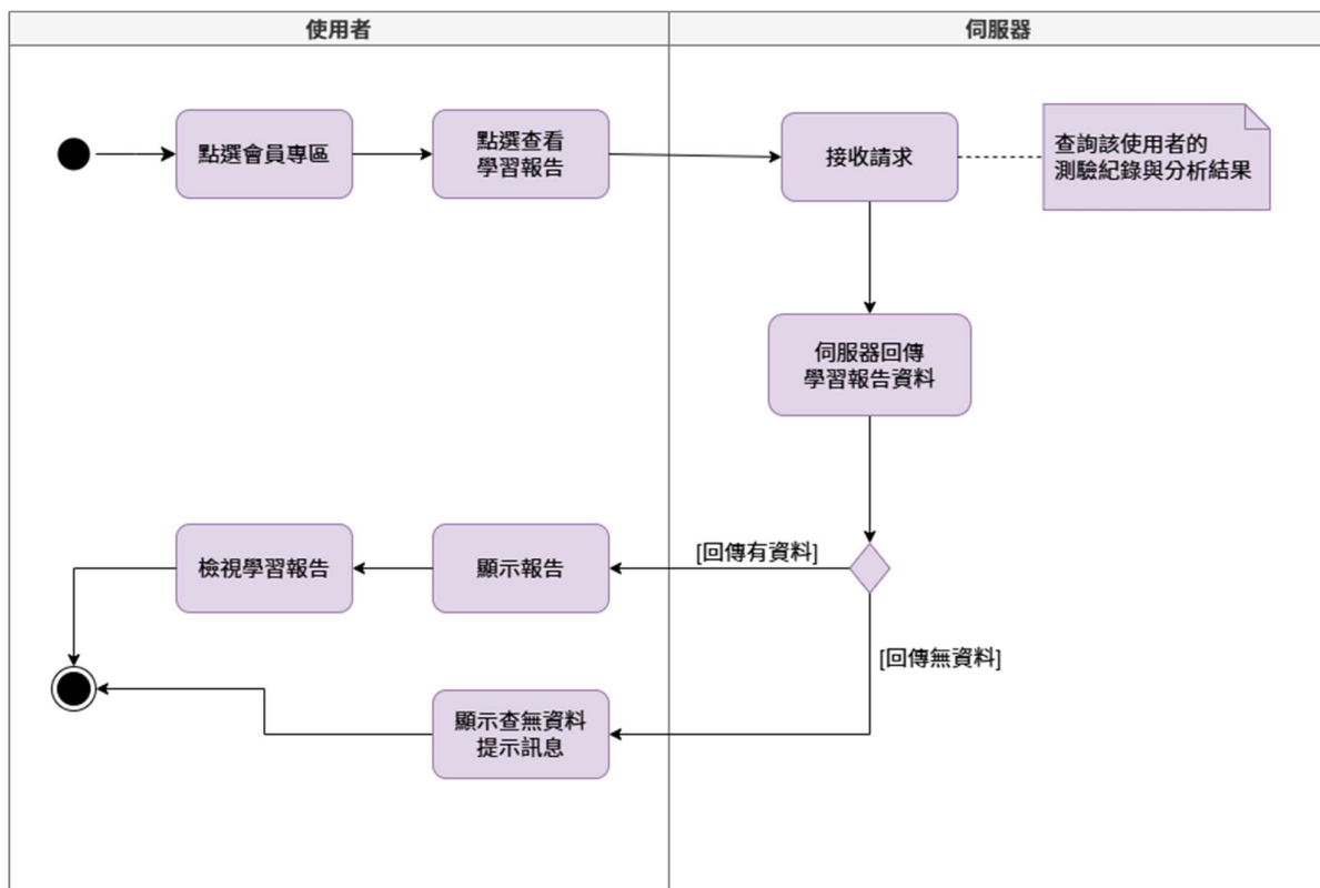
圖 5-3-6 查看學習歷程之活動圖
