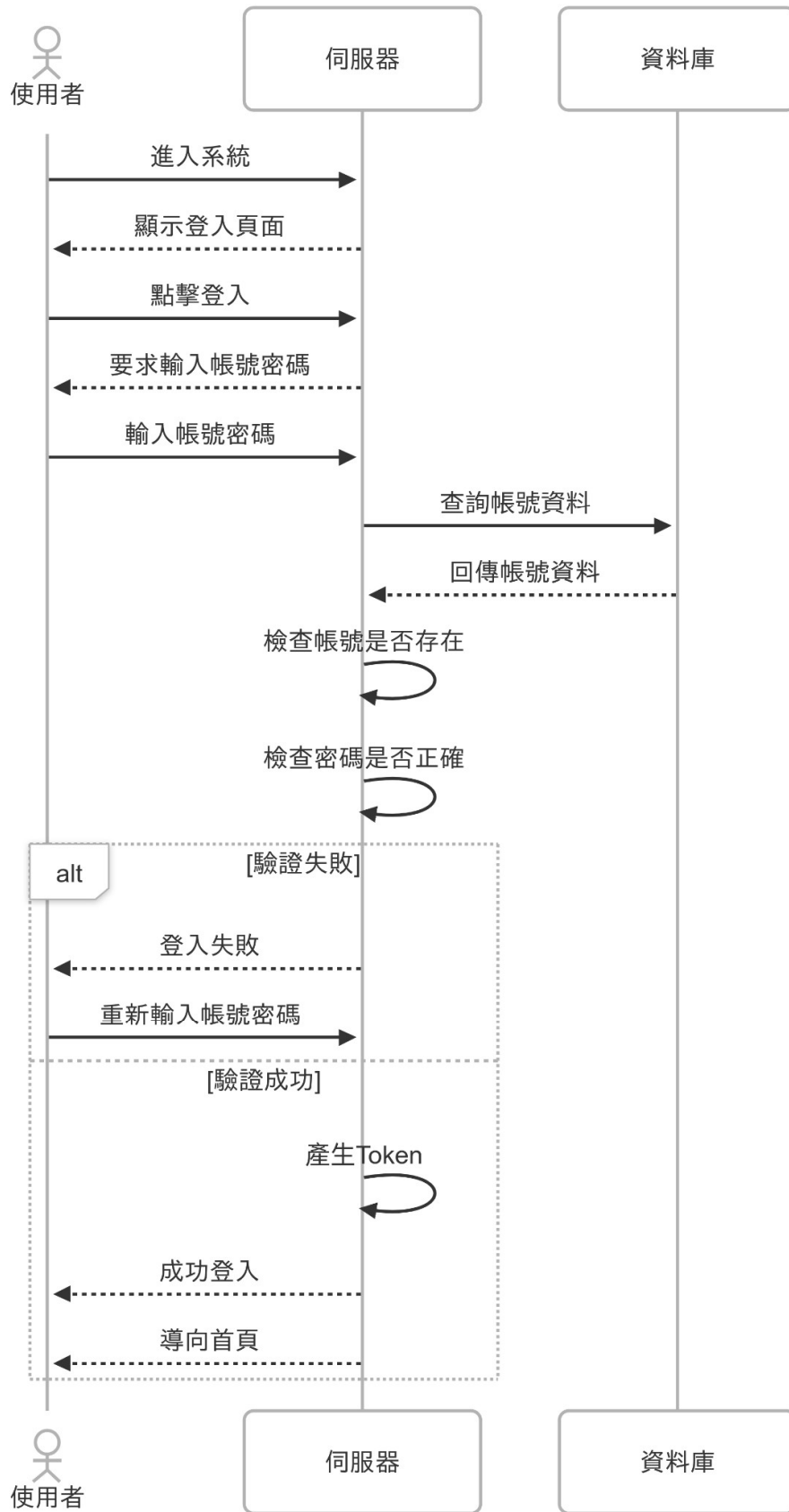
圖 6-1-2 登入之循序圖
