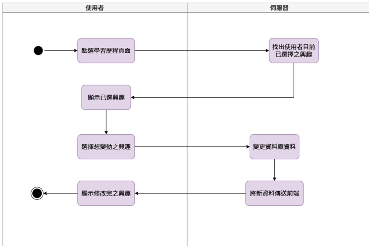
圖 5-3-11 選擇興趣之活動圖
