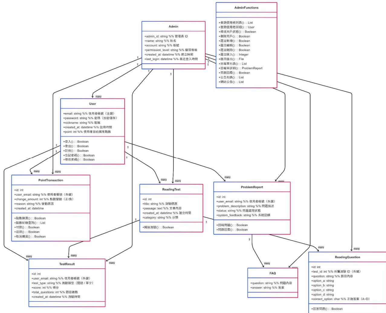
圖 5-4-1 分析類別圖
