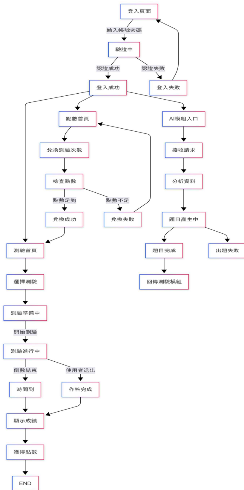
圖 7-4-1 狀態機
