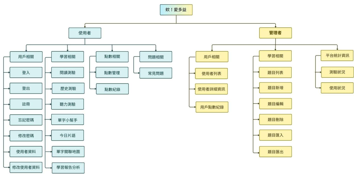
圖 3-1-1 系統架構圖
