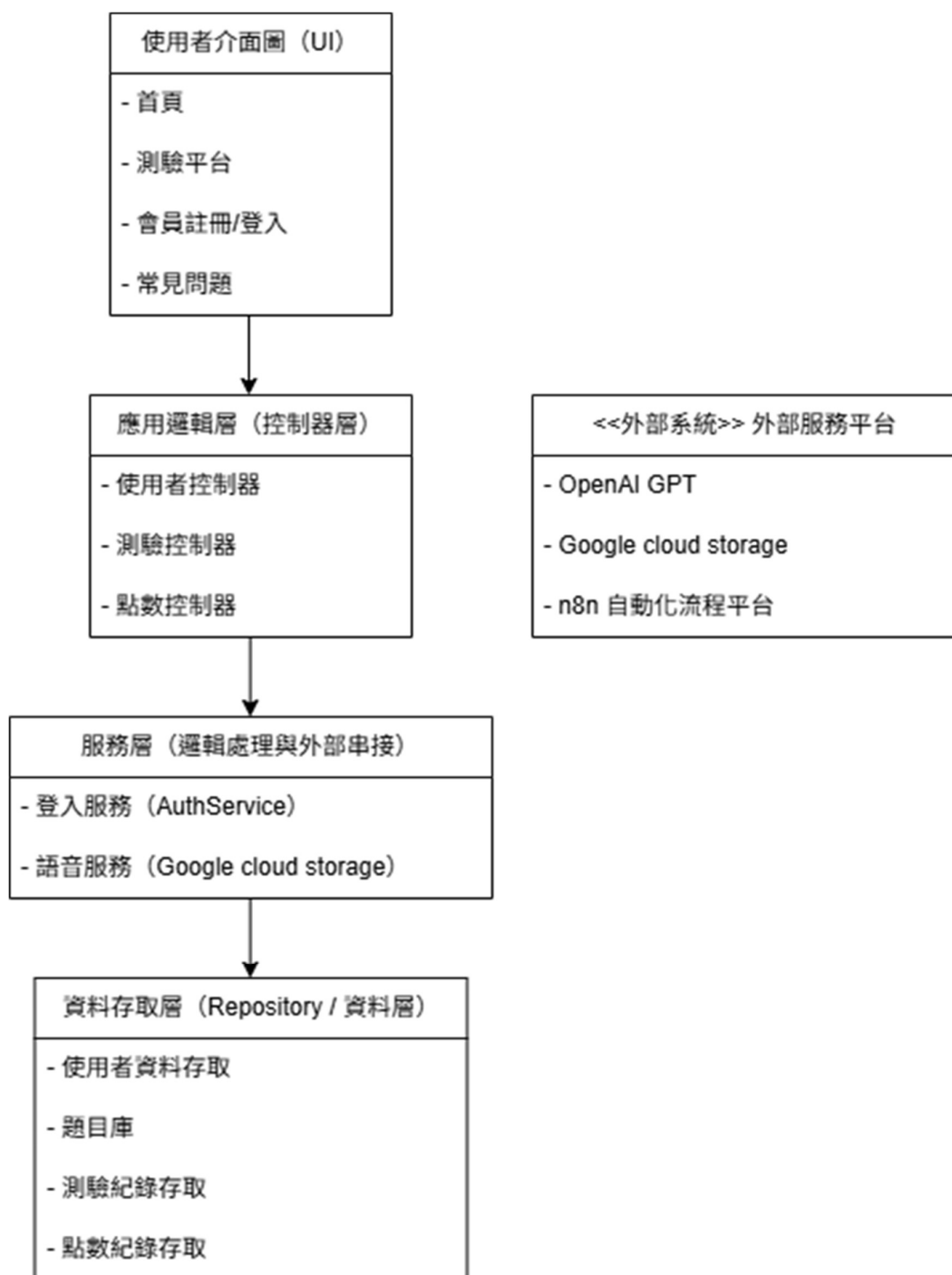
圖 7-2-1 套件圖
