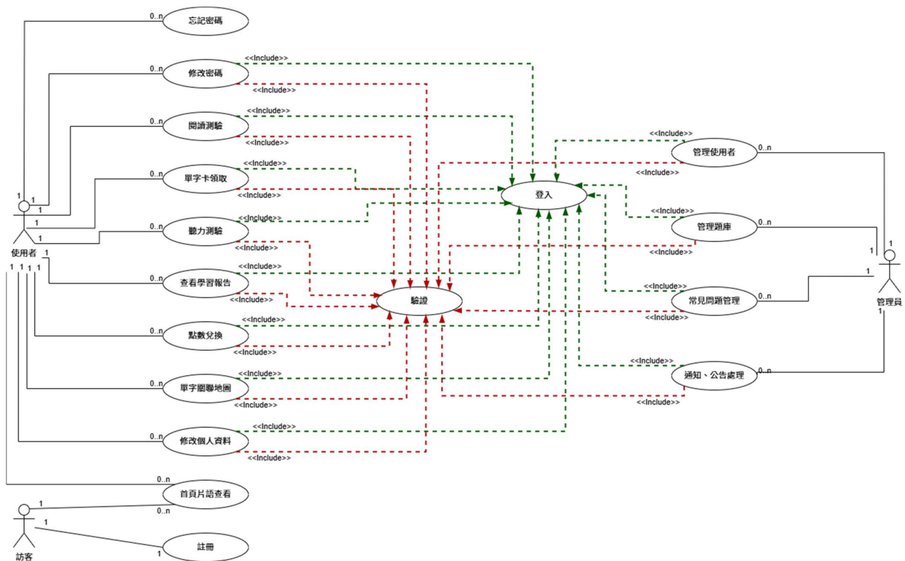
圖 5-2-1 使用個案圖
