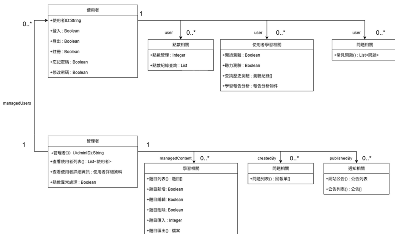
圖 6-2-1 設計類別圖
