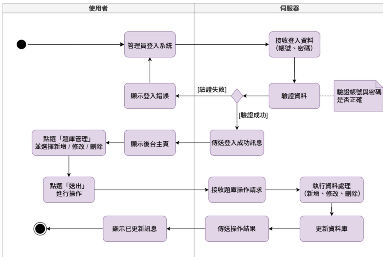
圖 5-3-7 管理員管理題庫之活動圖
