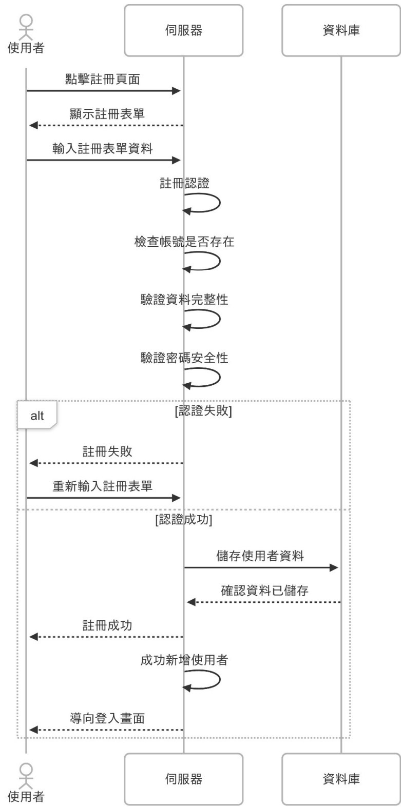
圖 6-1-1 註冊之循序圖
