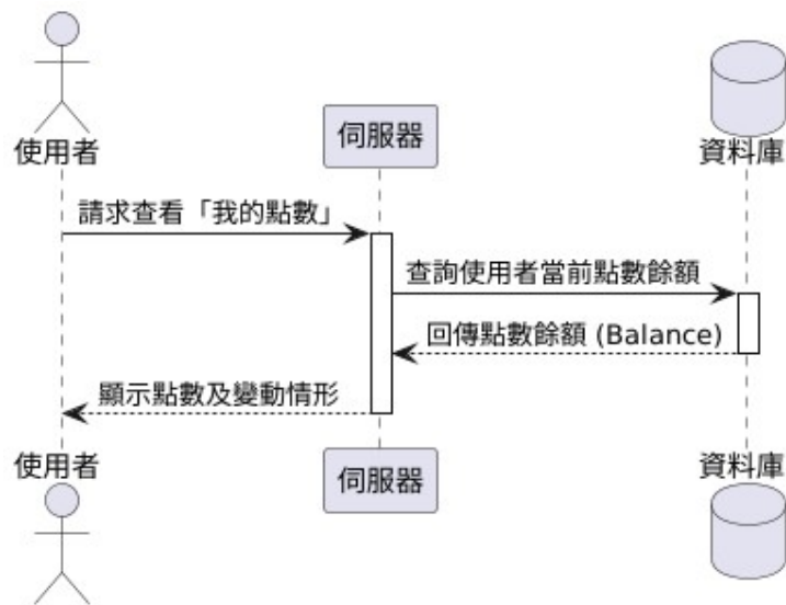
圖 6-1-12 點數變動查詢之循序圖
