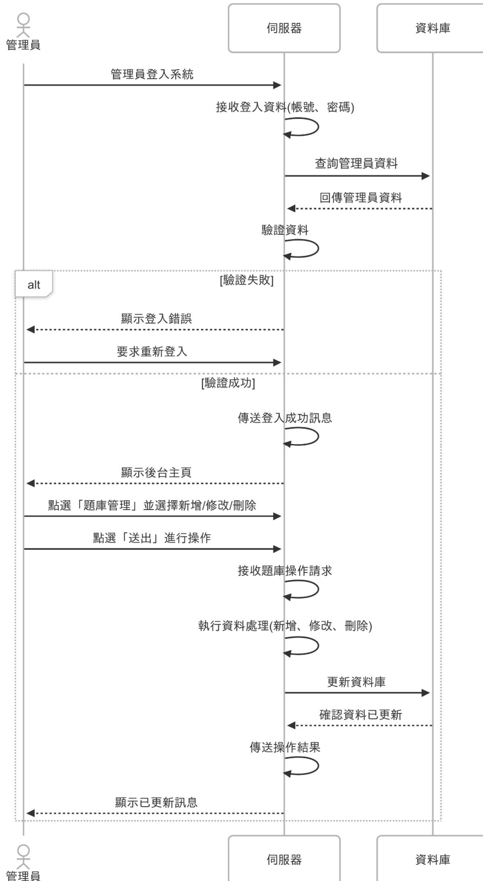
圖 6-1-7 管理員管理題庫之循序圖
