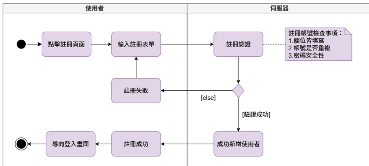
圖 5-3-1 註冊之活動圖
