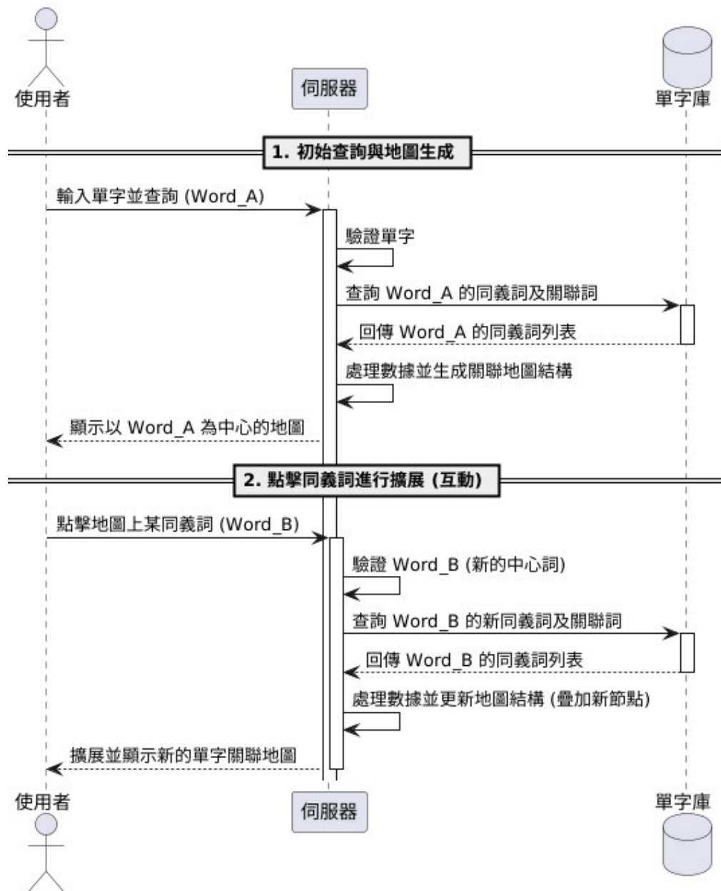
圖 6-1-10 單字關聯地圖之循序圖
