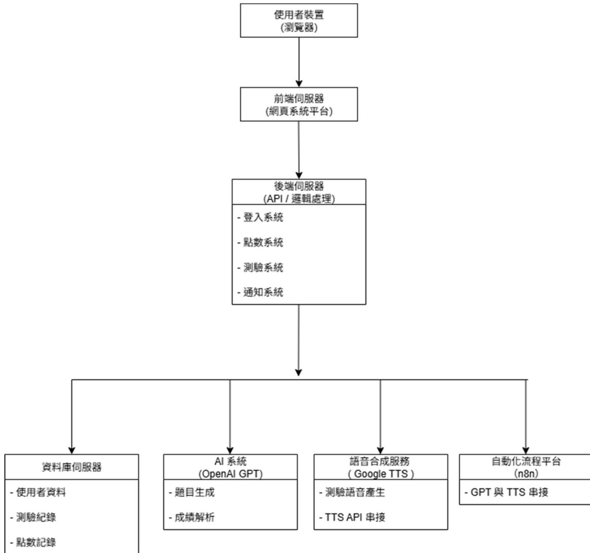
圖 7-1-1 佈署圖
