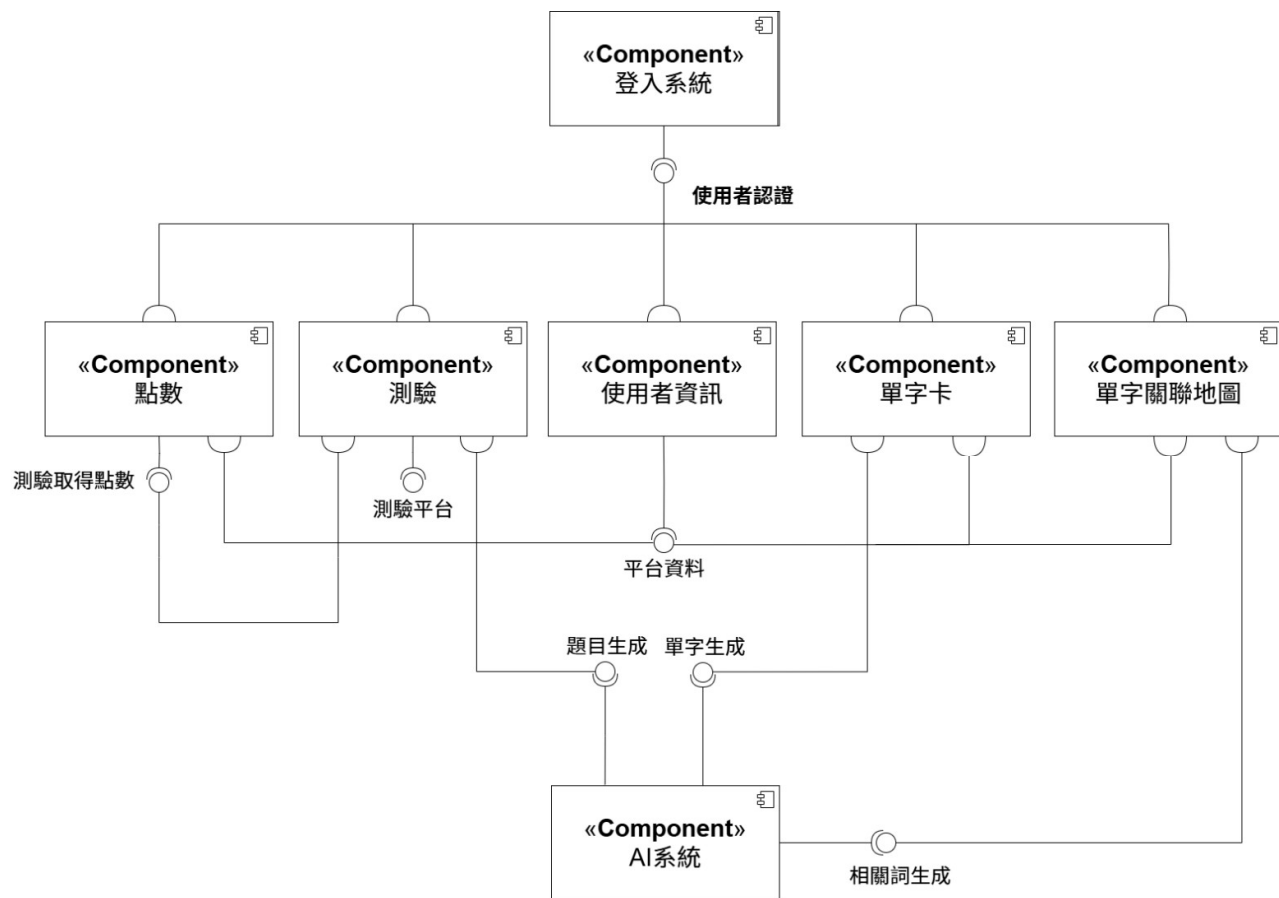
圖 7-3-1 元件圖
