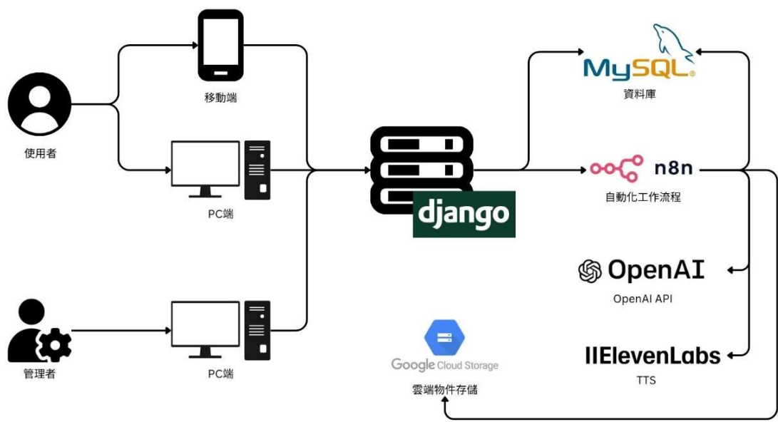
圖 3-1-1 系統架構圖
