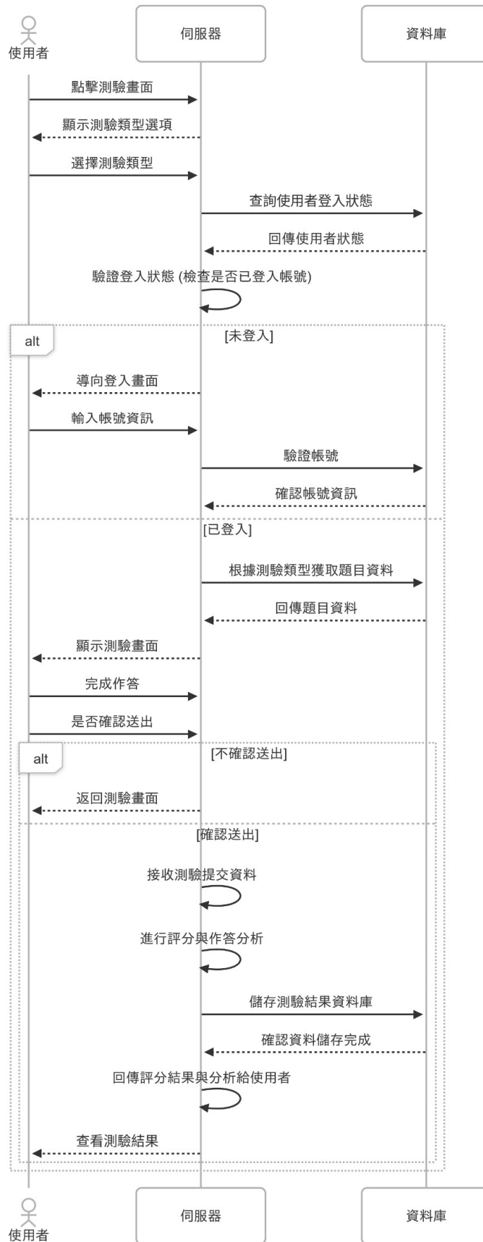
圖 6-1-5 測驗之循序圖
